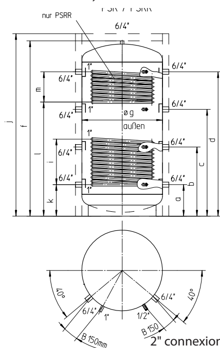
PSR/PSRR - Réservoir d'accumulation avec tuyauterie
