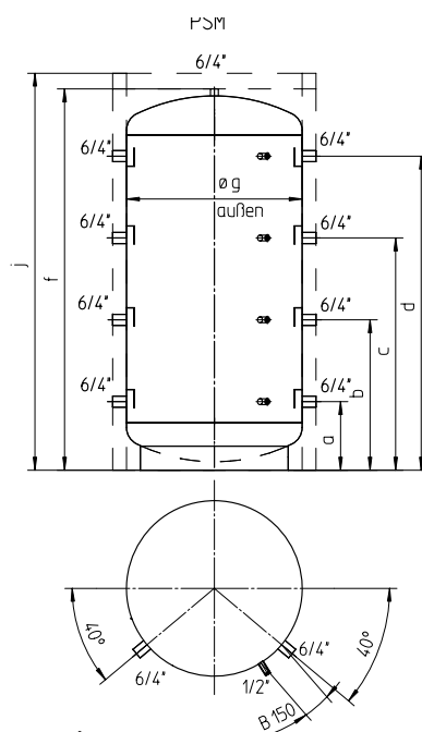
PSM - Réservoir d'accumulation
