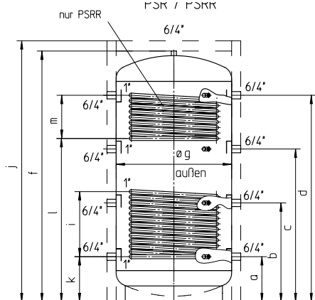
PSR/PSRR – Zalogovnik s cevnim toplotnim prenosnikom
