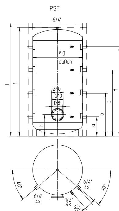
PSF - Pufferspeicher mit Flansch D 240
