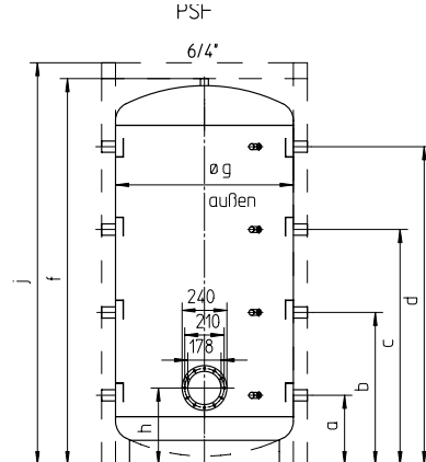
PSF – Zalogovnik s prirobnico D 240
