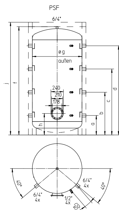
Zbiornik buforowy PSF z kołnierzem D 240
