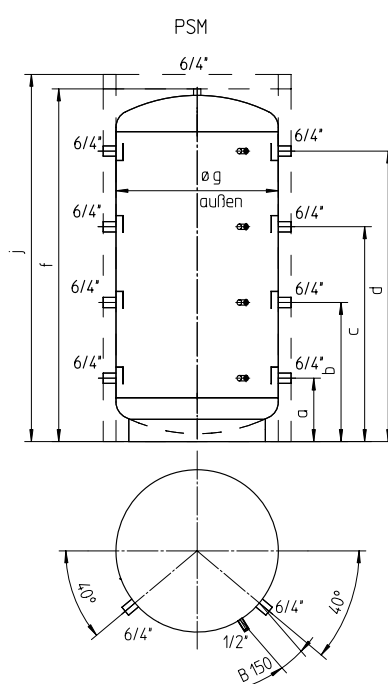
PSM - Pufferspeicher
