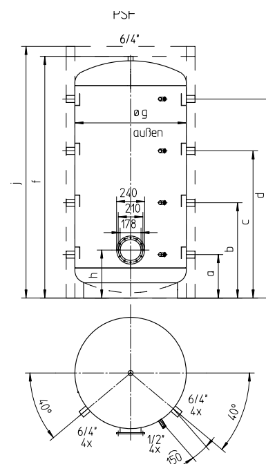
PSF - Réservoir d'accumulation avec bride D 240
