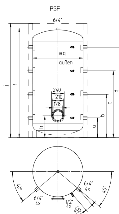
PSF - Bufferreservoir met flens D 240
